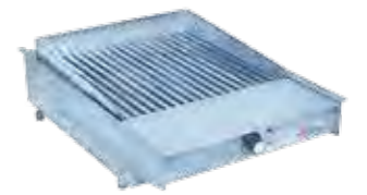
27061 Elektrischer Grill 230 V - 3,6 kW 40 x 60 cm H 15 cm Aufwärmzeit : 5 min T° regulierbar zwischen 50 und 320°C Gewicht 13 kg
