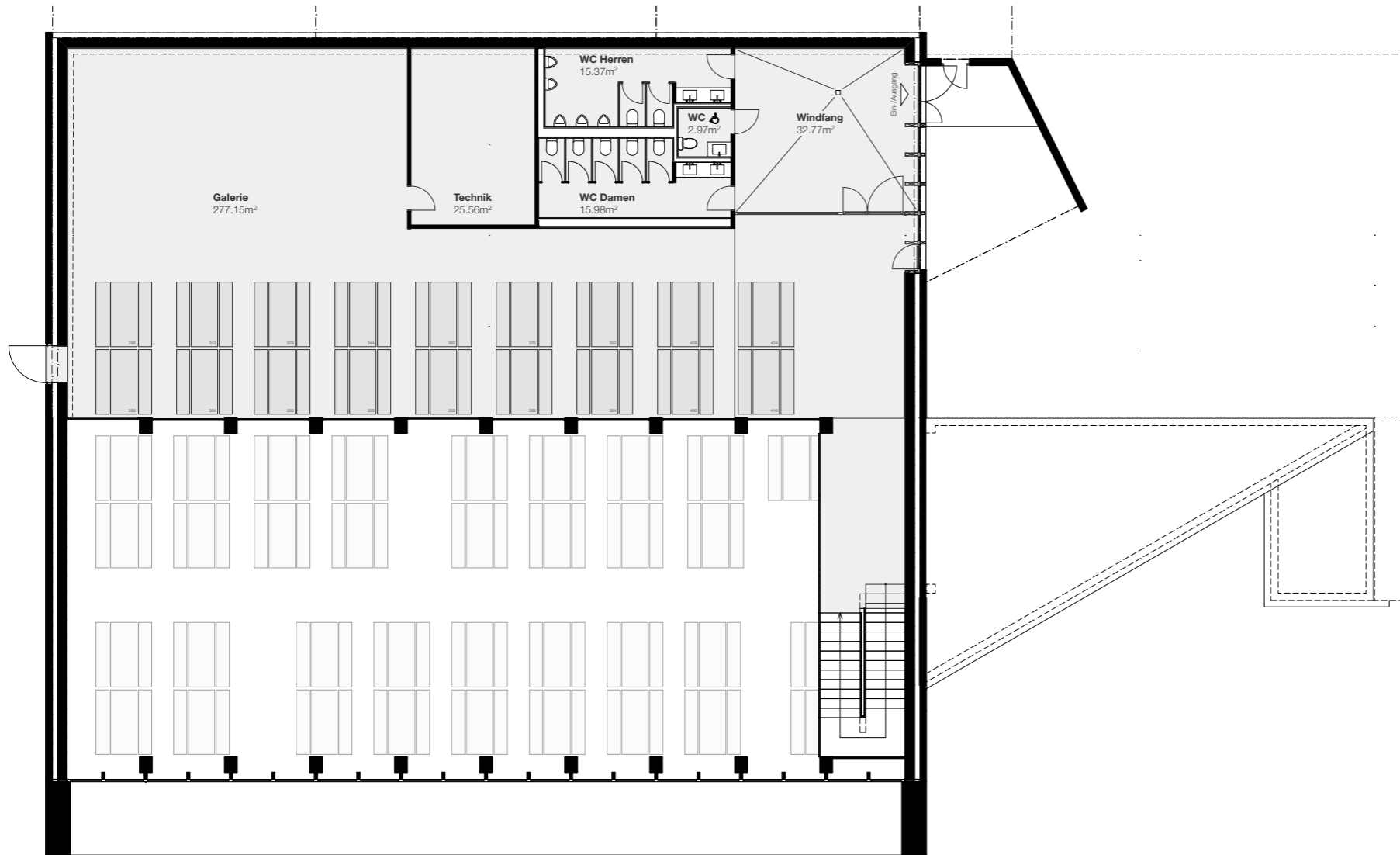
Obergeschoss
